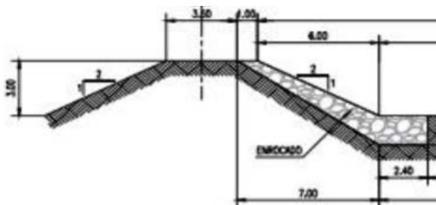
Figura 3: Sección típica de defensas ribereñas
