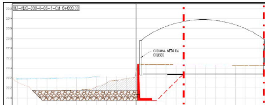
Figura N°5 Sección Alternativa 01
